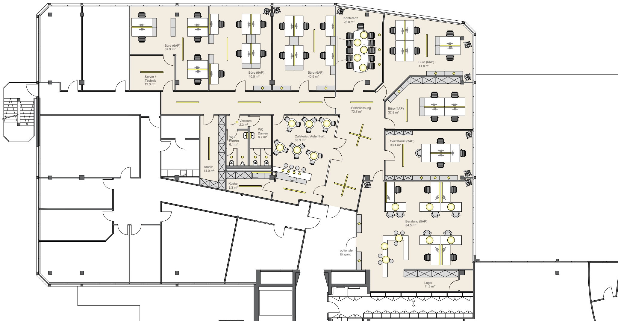
5509 Silver Cube Urdorf - Beleuchtungskonzept mit TW - 4.Obergeschoss - Büroraum 01-0401 (05_201218)
